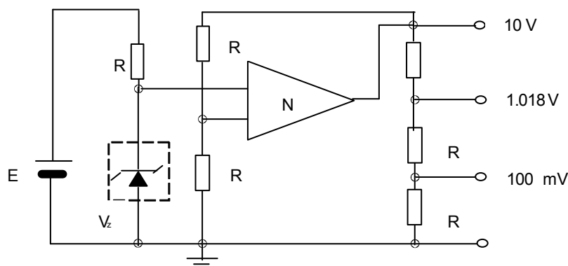
图 1 固态电压标准原理图
