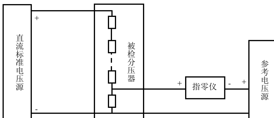
图 B1 参考电压法接线图
