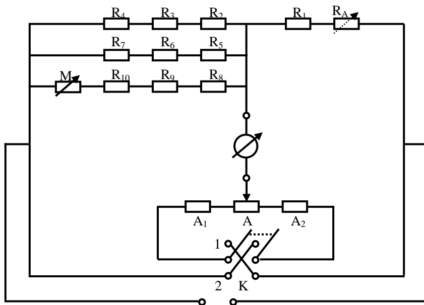
图 B2 哈蒙分压器校准接线图
