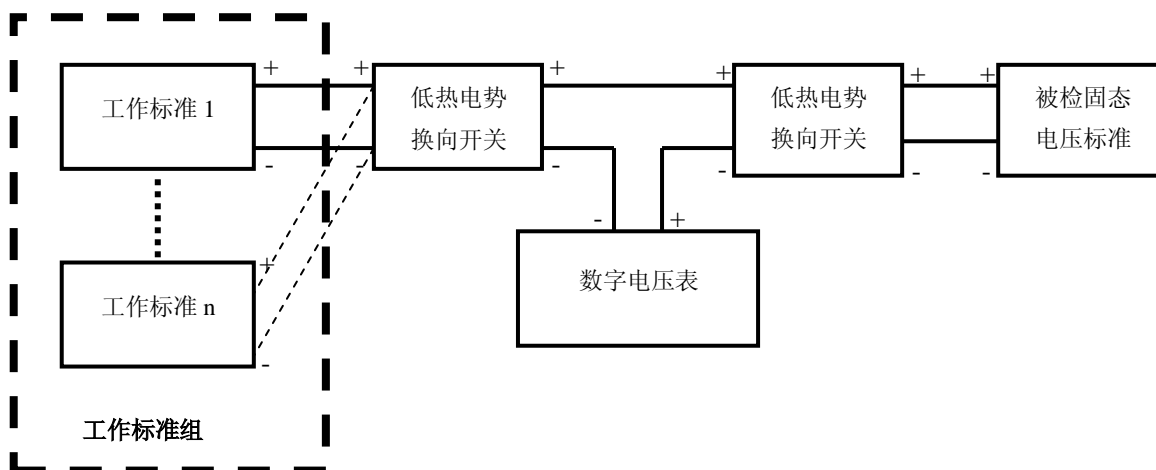
图3 工作标准组差值法检定固态电压标准
