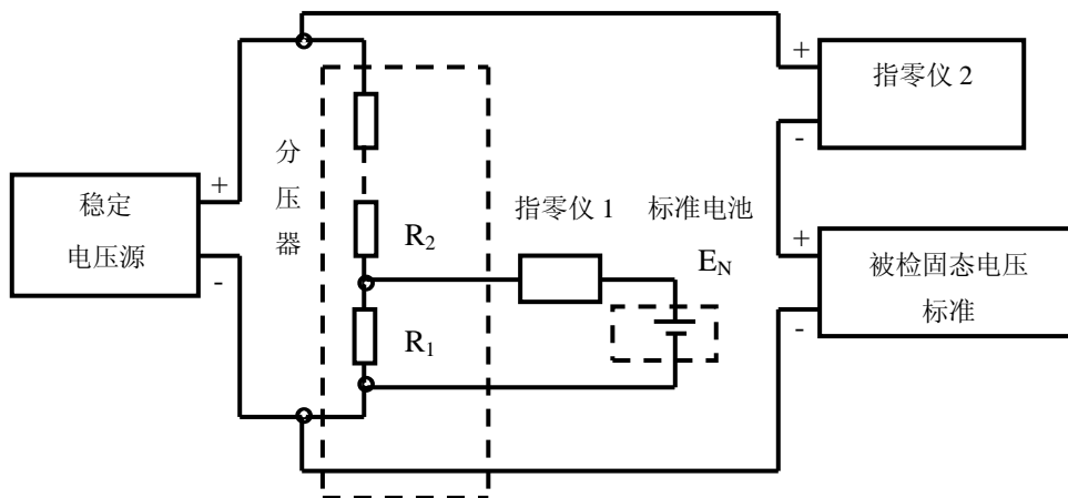
图 5 标准电池法检定固态电压标准的原理框图
