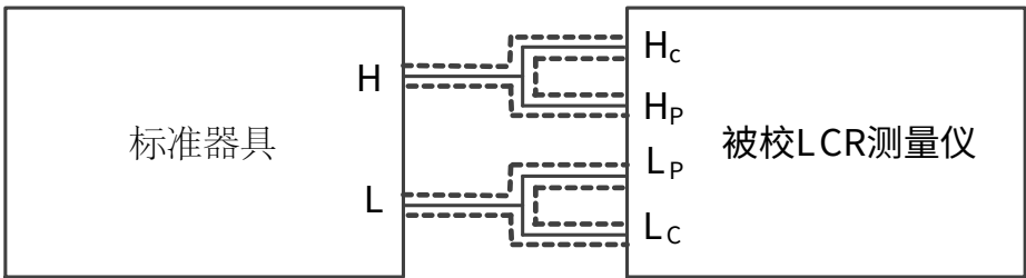
图 3 三端口结构标准器连接示意图
