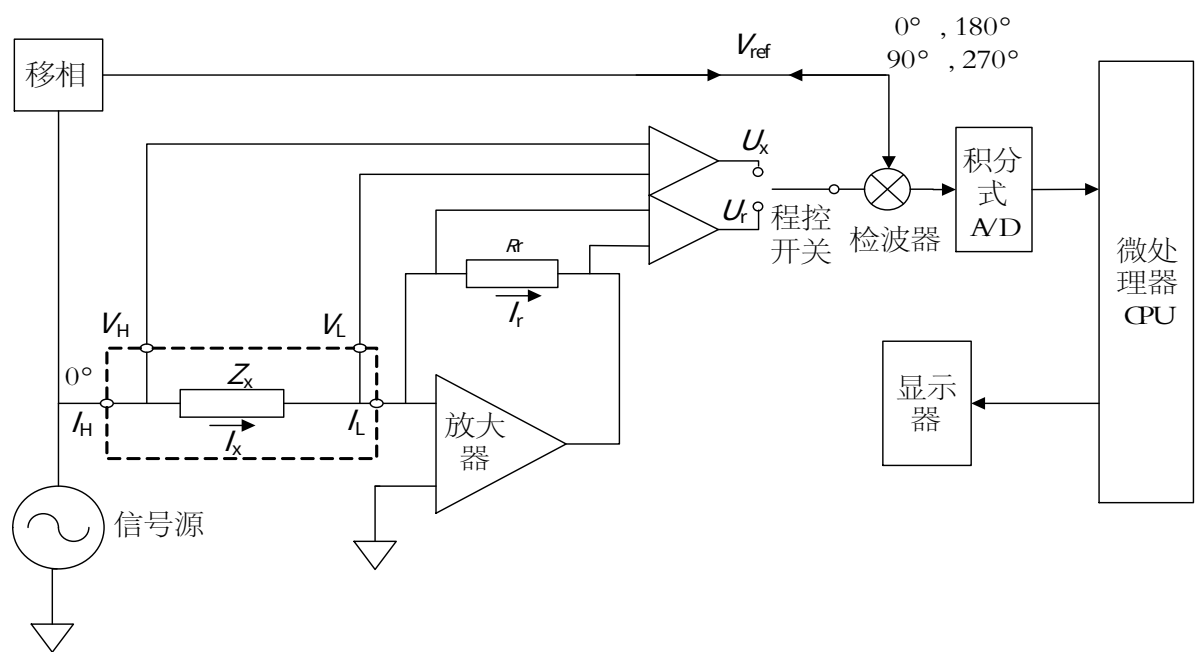
图 1 电压矢量比例法 LCR 测量仪测量原理图
