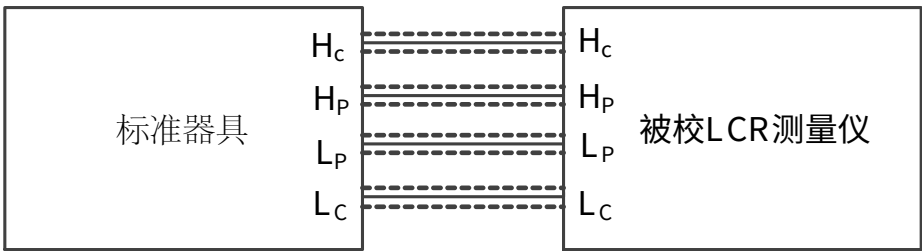
图 2 四端口结构标准器连接示意图
