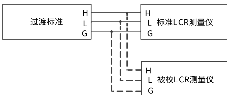
图 5 替代测量法连接示意图
