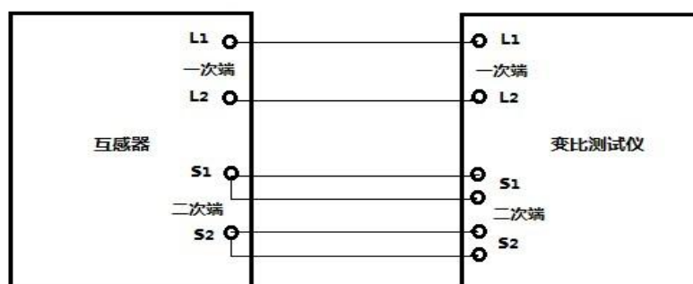
图 1 变比测试仪工作原理图框图
