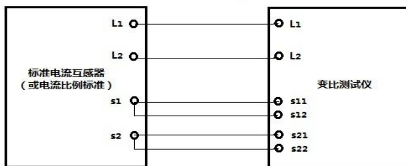
图 3 电流比较校准接线图
