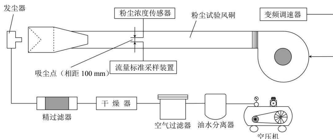
图1 粉尘试验风洞试验系统
