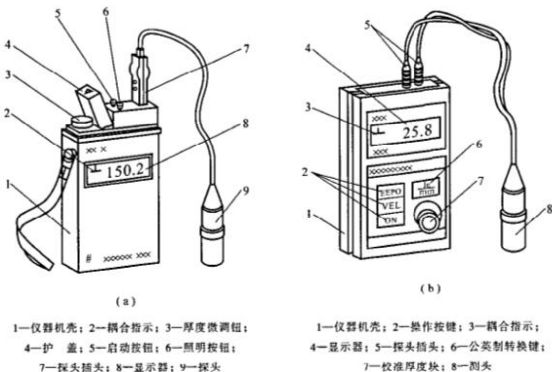
图1 仪器外形图
