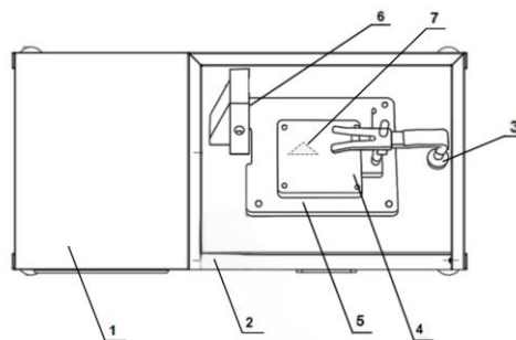
2固氧仪设备俯视图
