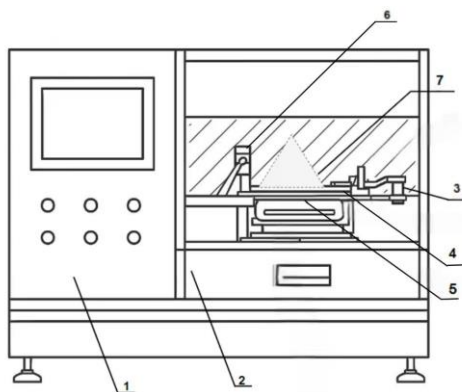
图1 固氧仪平面示意图
